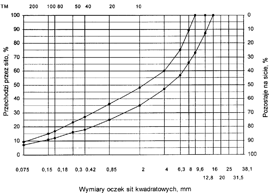
Rys. 1. Krzywe graniczne uziarnienia mieszanki mineralnej BA od 0 do 12,8 mm do warstwy ścieralnej nawierzchni drogi o obciążeniu ruchem KR3
