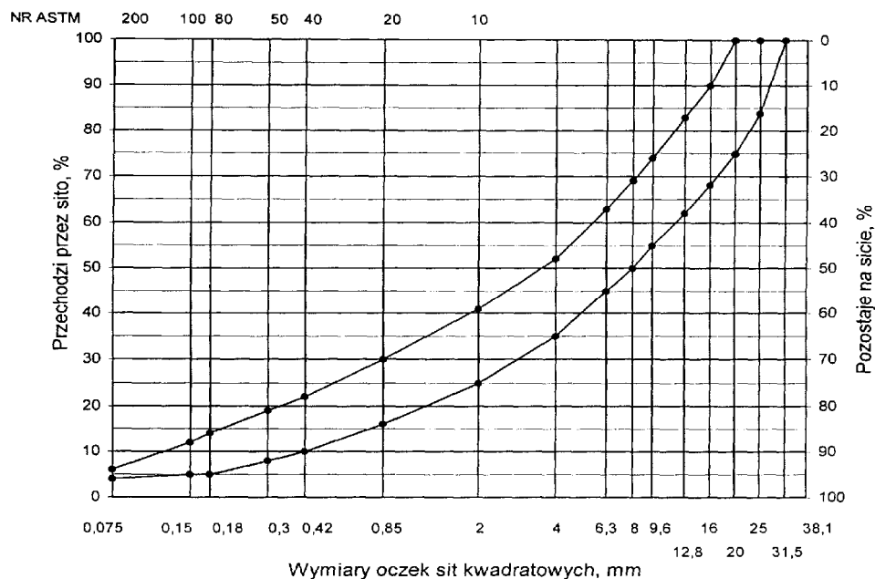
Rys. 2. Krzywe graniczne uziarnienia mieszanki mineralnej BA od 0 do 20 mm do warstwy wiążącej, wyrównawczej i wzmacniającej nawierzchni drogi o obciążeniu ruchem KR3
