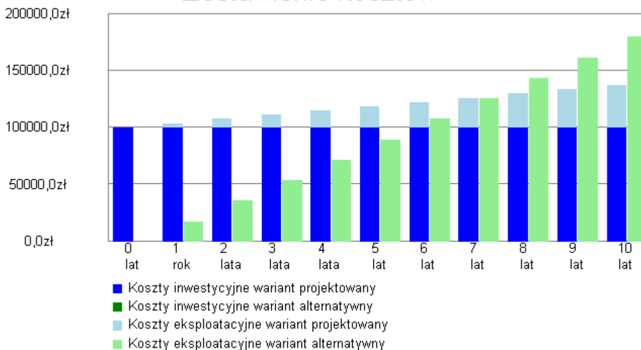
Wykres zestawienia kosztów inwestycyjnych i eksploatacyjnych za okres 10,00 lat
