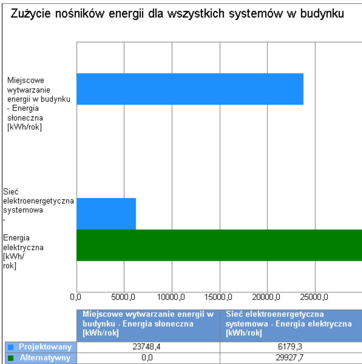
Wykres porównawczy zużycia nośników energii dla wszystkich systemów w budynku 11. Obliczenia optymalizacyjno-porównawcze kosztów eksploatacyjnych i inwestycyjnych systemu ogrzewania i wentylacji
