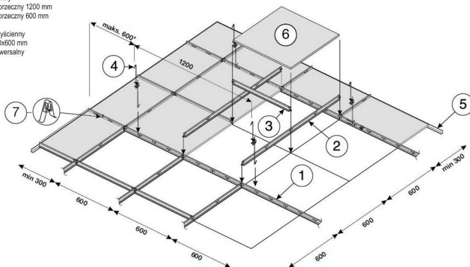
SCHEMAT SYSTEMU ZAWIESZENIA - SUFIT KASETONOWY
